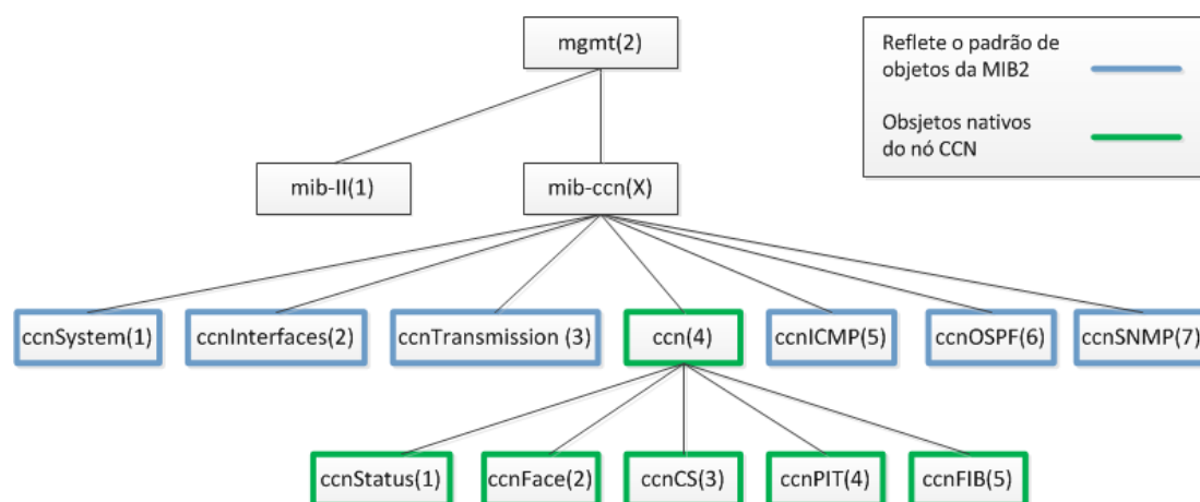
Figura 4: A MIB CCN e sua sub-árvore.
