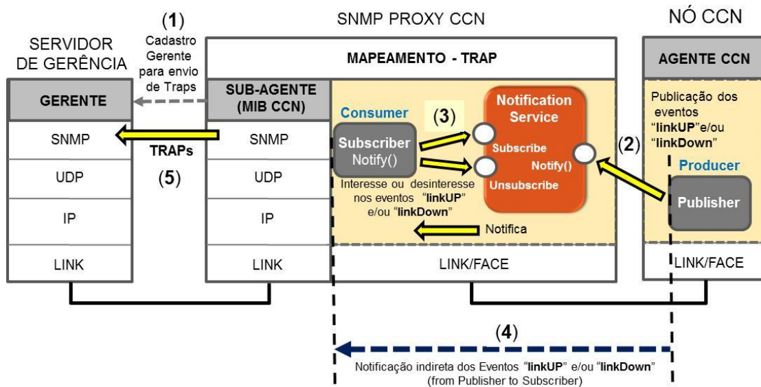
Figura 7: Arquitetura “Publishe/Subscribe Event Notification” para o SNMP Proxy CCN.
