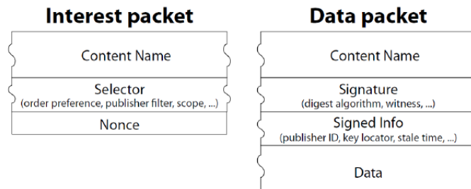
Figura 1. Pacote do CCN (reproduzido de [2]).
